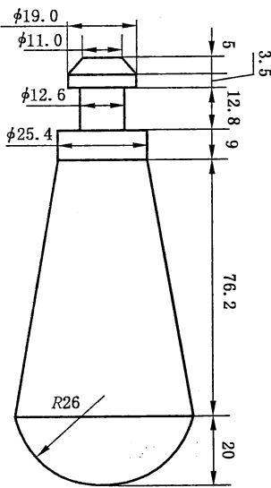
图 20 茄形锤
