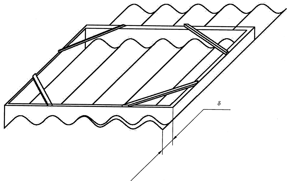
图 10 方正度试验
