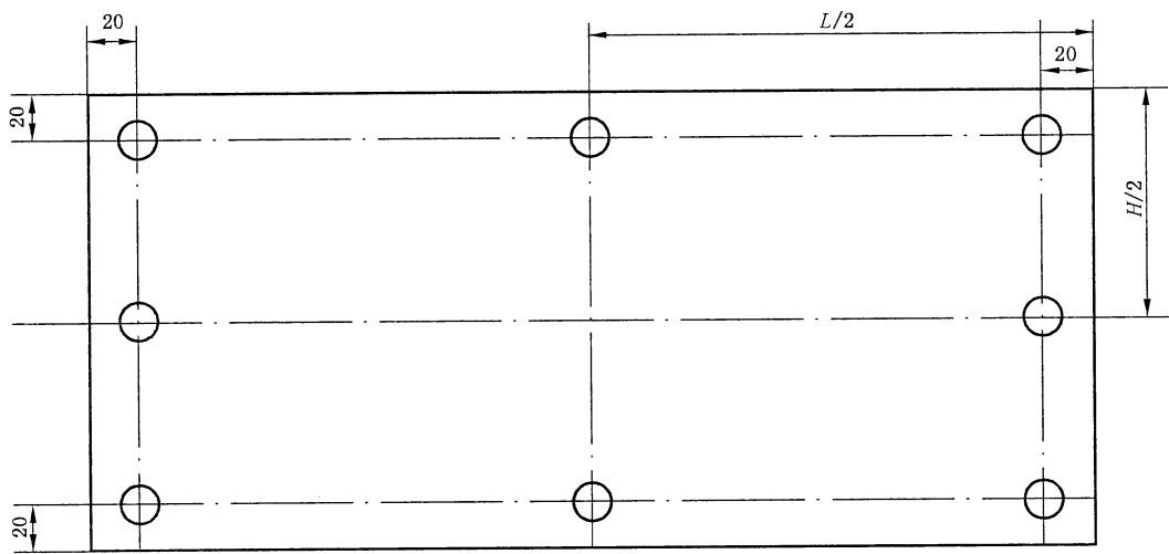
图 4 厚度不均匀度测量位置图
