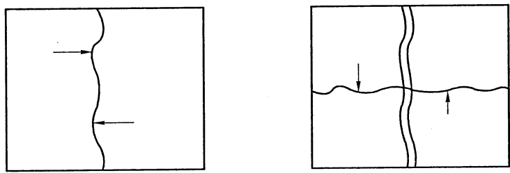
图 17 平板抗折试验断裂处厚度测量位置
